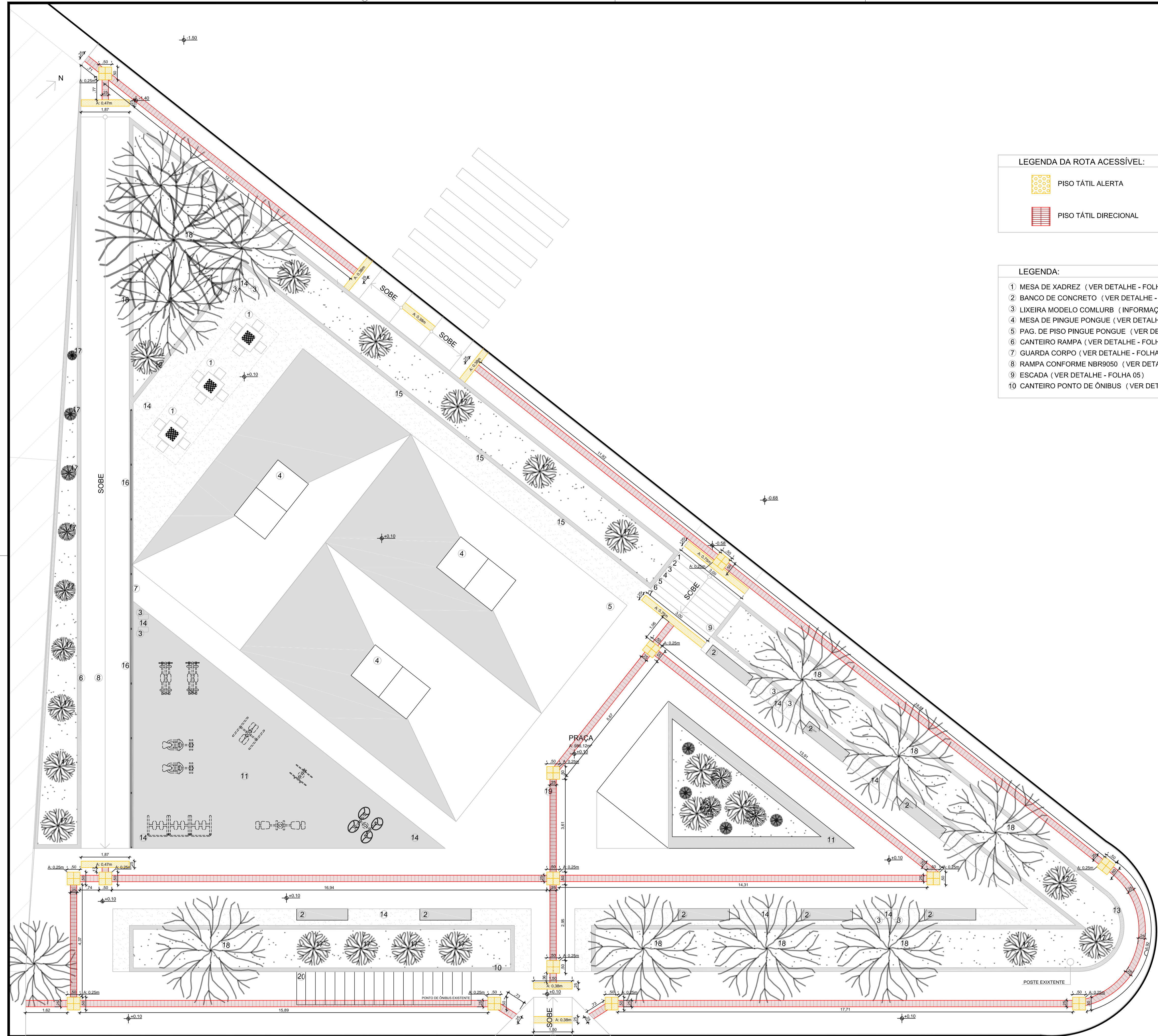
PLANTA BAIXA - ROTA ACESSÍVEL ESCALA 1:75
